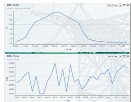
Коэффициент нелинейных искажений тока (THDi) и коэффициент нелинейных искажений напряжения (THDv) активного фильтра подавления гармоник (вход или нагрузка)
