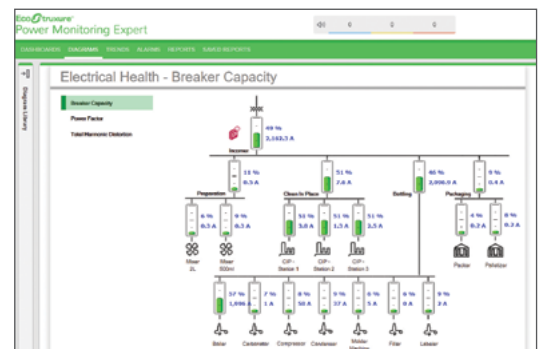
Схема состояния электросети
