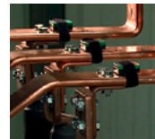
Комплект датчиков Easergy TH110, установленных на 3 фазах электрического соединения
