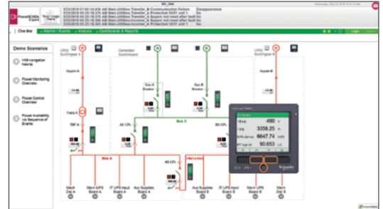
Принципиальная схема электрической сети (с цветовой анимацией)
