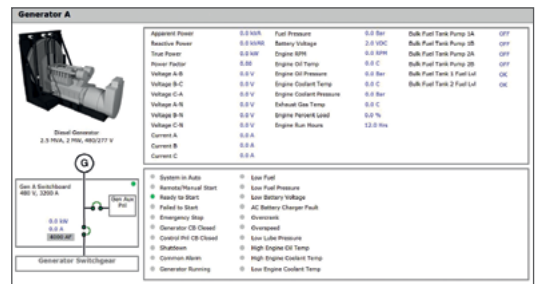
Схема генератора
