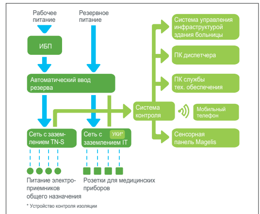
Функциональная схема распределительного щита операционной
