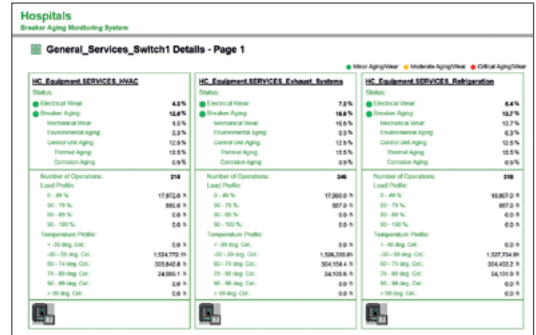
Схема старения автоматических выключателей
